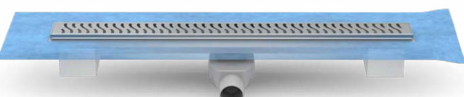
Lineární plastový žlab D50 s izolací, nerezovým rámečkem a otočným sifonem
